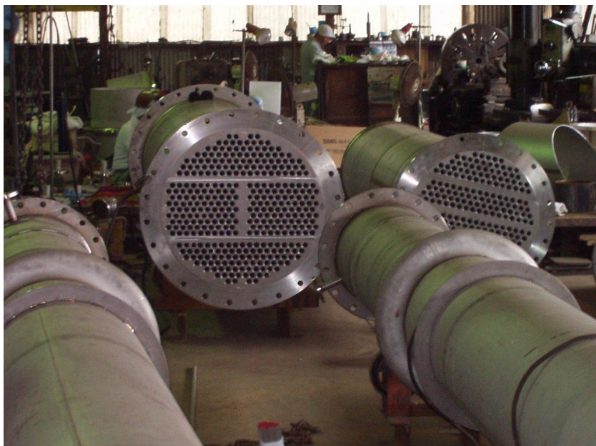
濃縮装置用加熱缶
