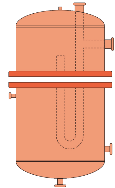
2分割型NEW貯湯槽
